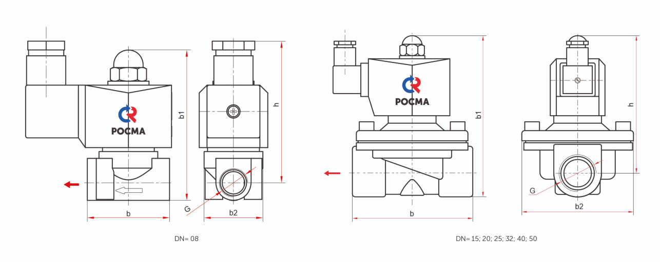
Габаритные и присоединительные размеры (мм), вес (кг)
